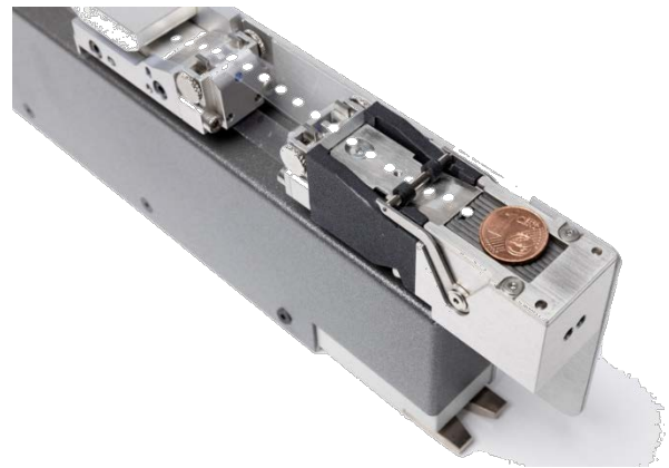
Zuführung eines Sensors von 3 mm Durchmesser
